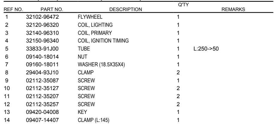
FIG.303A (1-E-2) MAGNETO (DT25K P36)
